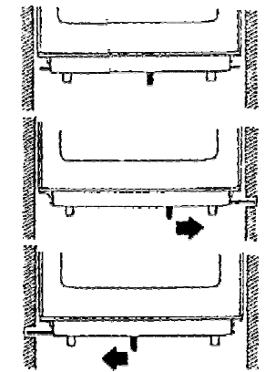
Abb. Stabilisatorriegel
